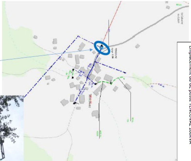
Emplacement du GE poste TENCOVAZ 100KVA
